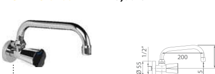
Con florón Ø 55 mm With Ø 55 mm flange
